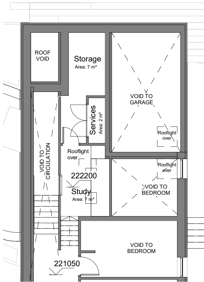
2 Mezzanine Plan 1 : 100
